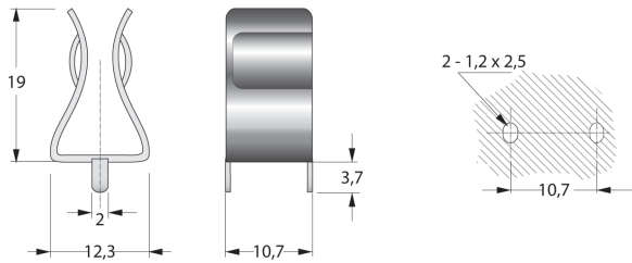
PINZE PER FUSIBILI 10x38 0900502 FUSE CLIPS FOR FUSES 10x38 0900502
