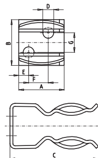
PINZE PER FUSIBILI 22x58 0900508 FUSE CLIPS FOR FUSES 22x58 0900508
