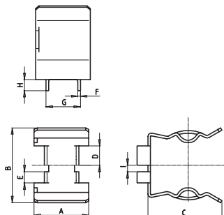
PINZE PER FUSIBILI 22x58 0900507 FUSE CLIPS FOR FUSES 22x58 0900507
