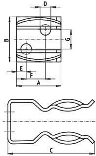
PINZE PER FUSIBILI 10x38 0900504 FUSE CLIPS FOR FUSES 10x38 0900504
